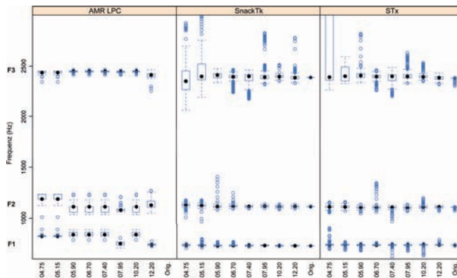
Abbildung 4: Formantmessungen in synthetisierten, stationären /a/-Vokal
