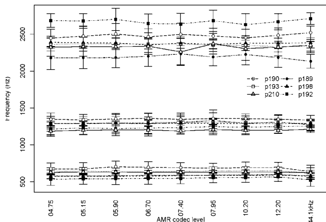
Abbildung 3: Manuell korrigierte Formantmessungen bei /a/-Vokalen von 6 Sprechern.
